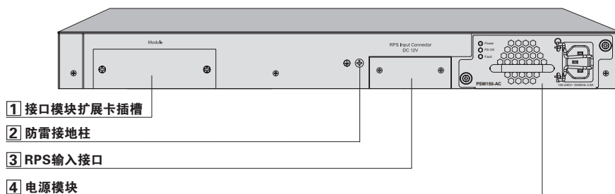
图1-2 T3700G-28TQ后面板示意图(1)
