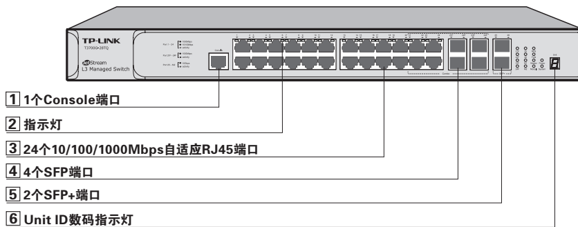
图1-1 T3700G-28TQ前面板示意图
